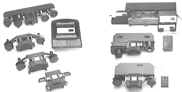
Modulare, leicht wechselbare Filmtransporte, manuell bedienbar, motorisch und automatisch. Modular film carriers and transports, manually operated, motorized or automatic, easy to exchange.
